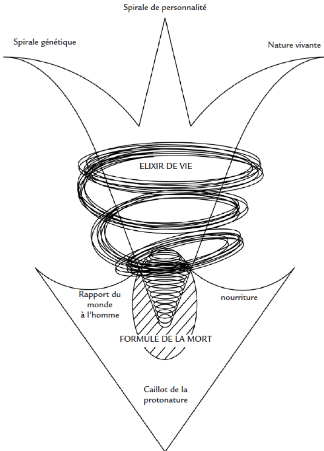
12-2. Interaction entre l'élixir de vie et la formule de la mort.
